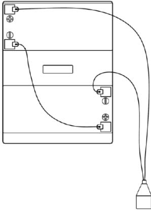
Рисунок 9 – Схема соединений АКБ в группе изделия SKAT BC 24/18S3 RACK исп.Л
